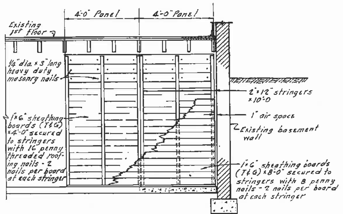
ELEVATION
